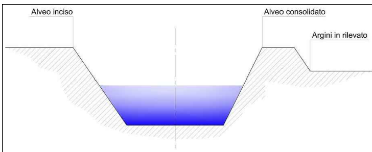
Sezione tipo di alveo fluviale con individuazione dei punti per la misurazione delle distanze
